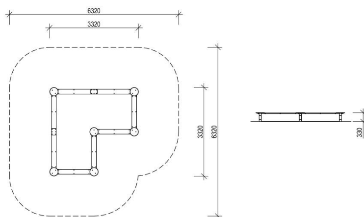
WYPOSAŻENIE OPCJONALNE ZE-207 Stolik do piaskownicy
