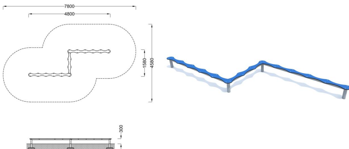
RZUT I ELEWACJA
