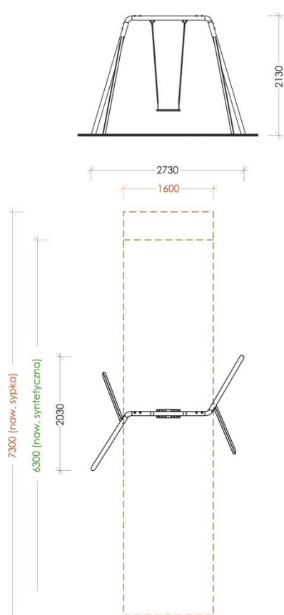
RZUT I ELEWACJA
