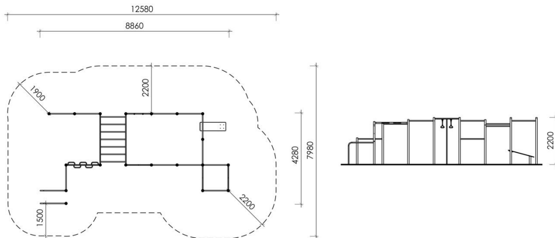
RZUT I ELEWACJA
