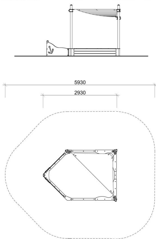
RZUT I ELEWACJA
